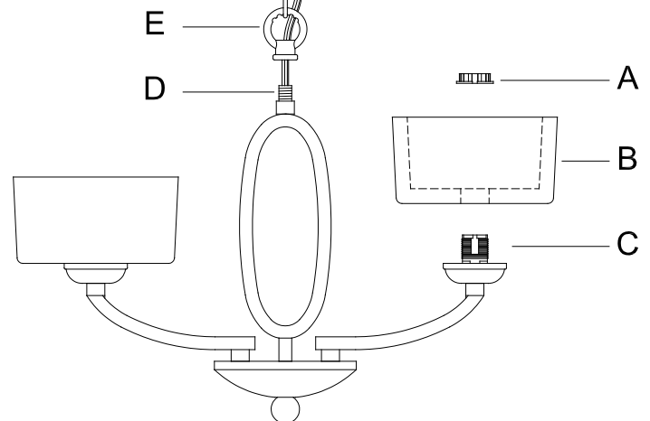
Chandelier
